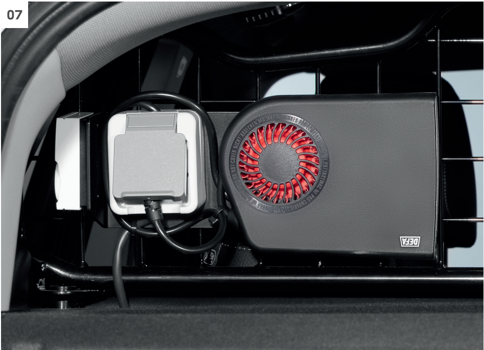
[ 05 / 06 ] Waffenkasten in Kofferraum (nur für BMW X1 und BMW 5er) [ 07 ] Heizlüfter inkl. Thermostat mit Versorgung im Gepäckraum; nur für X-Fahrzeuge erhältlich.
