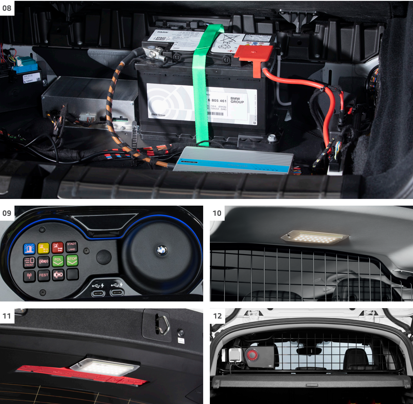
[ 08 ] Integrierte zweite Batterie im Gepäckraum zur zusätzlichen Energieversorgung. [ 09 ] Integriertes Schaltzentrum. [ 10 ] Zusätzliche LED-Gepäckraumbeleuchtung im Dachhimmel (nur in Verbindung mit LED-Gepäckraumbeleuchtung in der Heckklappe bestellbar) [ 11 ] LED-Gepäckraumbeleuchtung zur optimalen Ausleuchtung des Gepäckraums; Aktivierung über Heckklappenöffnung und separaten Schalter. [ 12 ] Gepäckraumtrenngitter zur Sicherung des Fahrgastraums.
