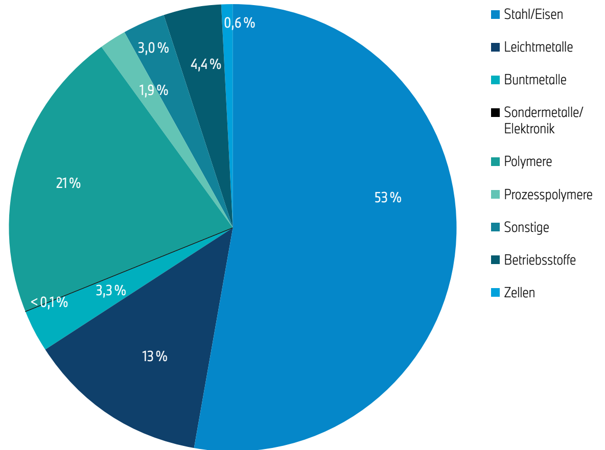
Abb. 2: Werkstoffzusammensetzung des BMW 120 zum Produktionsstart. Die angegebenen Werte können Rundungsdifferenzen aufweisen.
