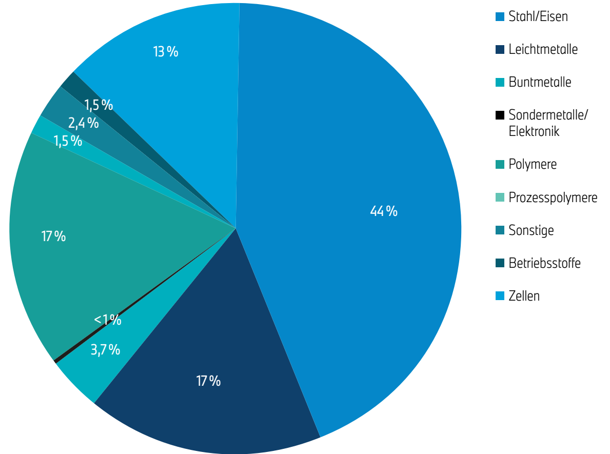
Abb. 2: Werkstoffzusammensetzung des BMW iX2 xDrive30 zum Produktionsstart. Die angegebenen Werte können Rundungsdifferenzen aufweisen.
